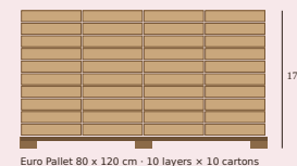
Euro Pallet 80 x 120 cm · 10 layers × 10 cartons
