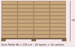
Euro Pallet 80 x 120 cm · 10 layers · 16 cartons
